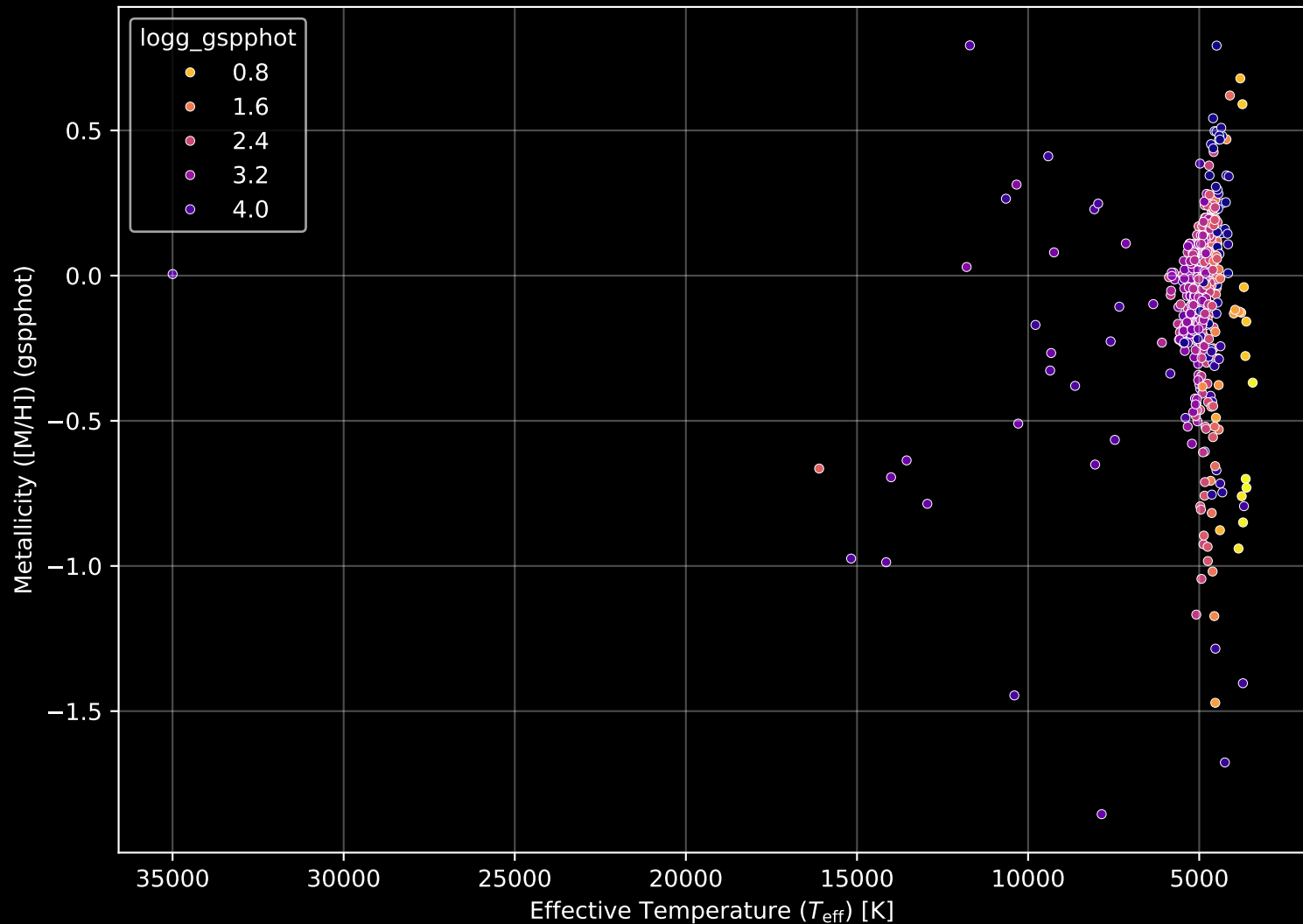
APOGEE DR17 Field: [100+12] Stellar Population Parameters (n= 547)
